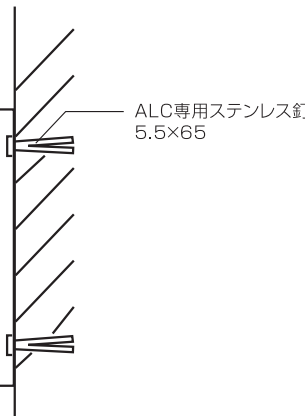
▶ALC 壁面へ取り付けの場合
