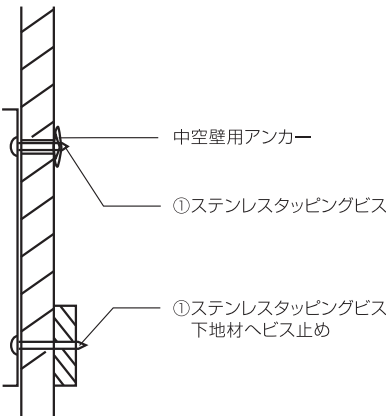
▶サイディング壁面へ取り付けの場合
