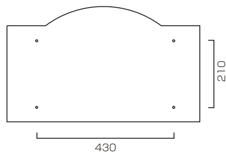
▼天アーチ：H360×W600mm
